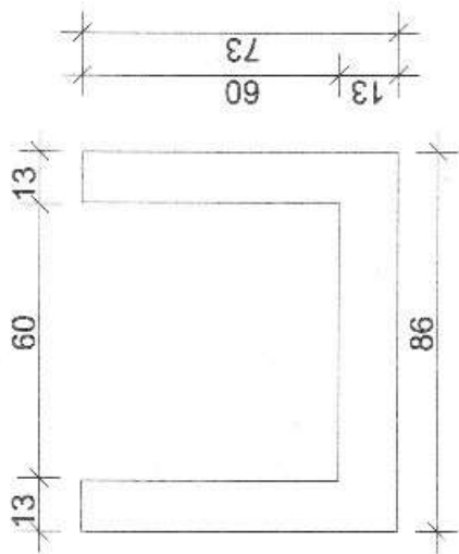
ПРЕСЕК 1-1
